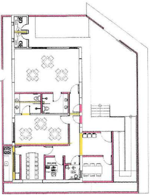
② PLANTA BAIXA - REFORMA
