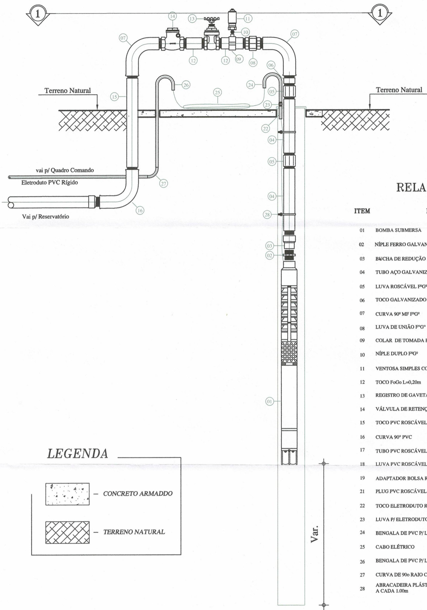
1 CORTE ESQUEMÁTICO A-A ESCALA 1:100
