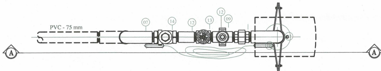
2 PLANTA BAIXA POÇO ESCALA 1:100
