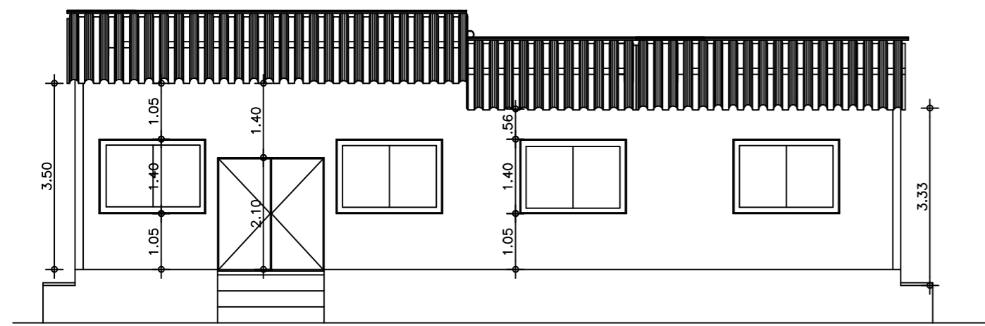
2 FACHADA ESC 1/100
