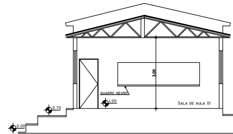
4 CORTE B ESC 1/100
