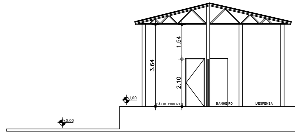
5 CORTE C ESC 1/100
