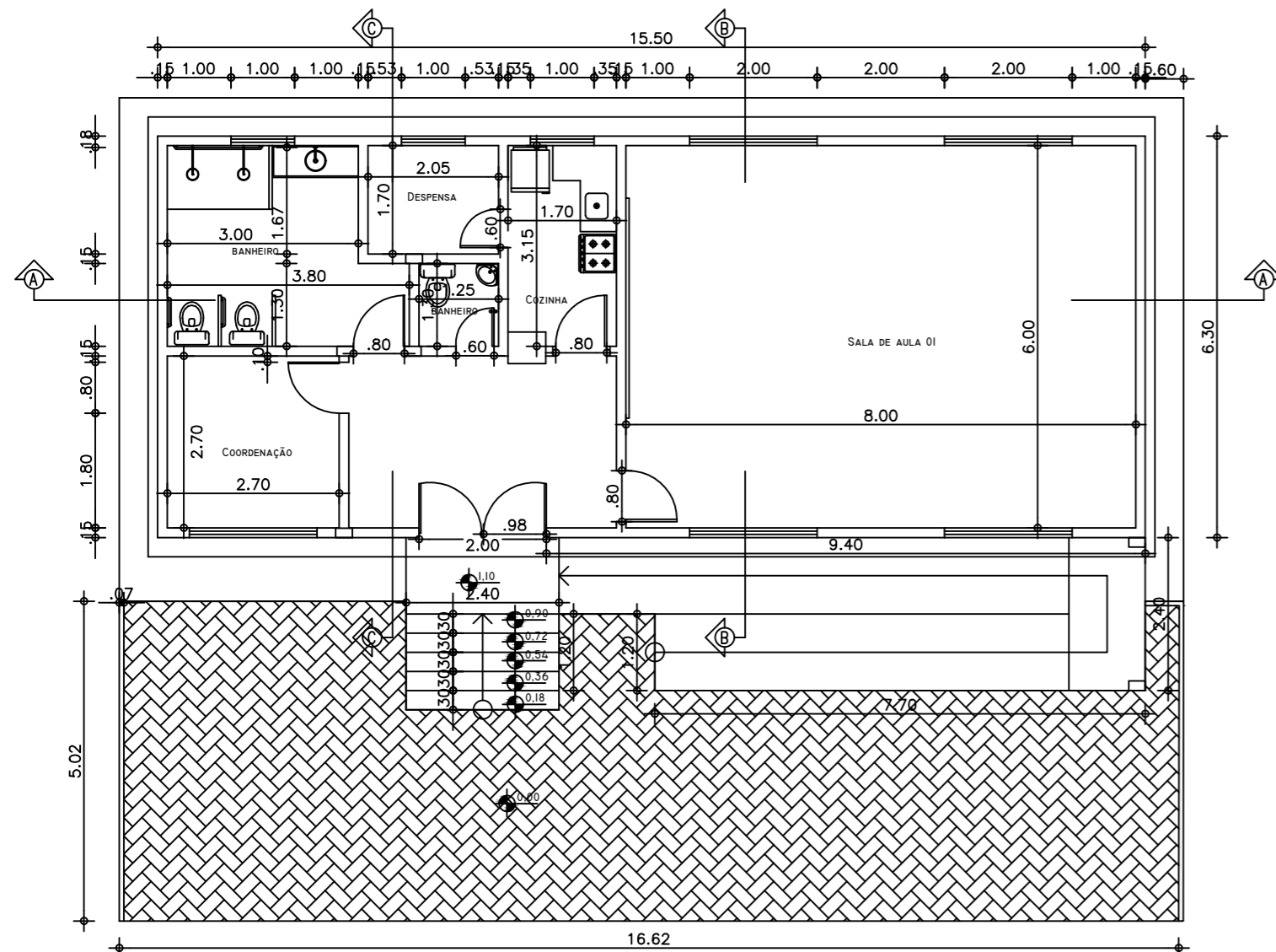
1 PLANTA BAIXA ESC 1/100
