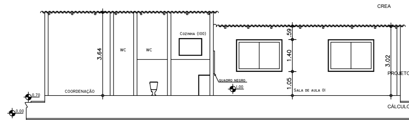
3 CORTE A ESC 1/100
