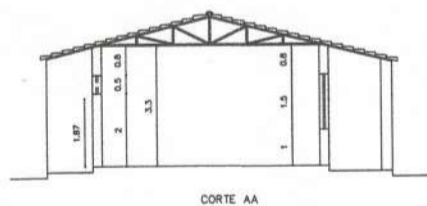
3 CORTE AA ESC 1/100
