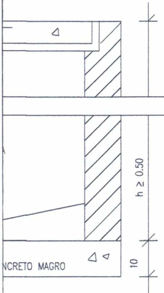
CORTE BB'
